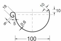
GRONDAIA "BOCCA" 10 cm TUBO PLUVIALE Ø 6 cm
